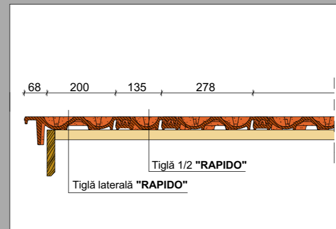
Montaj tigla laterala stanga
