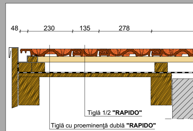
Montaj tigla laterala cu proeminenta dubla
