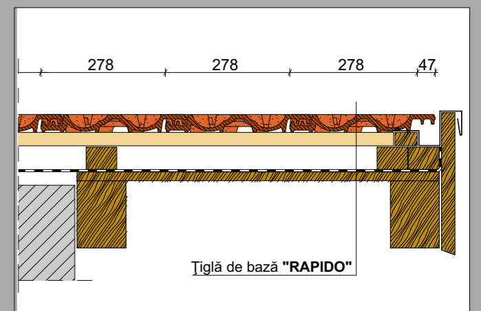
Montaj tigla de baza
