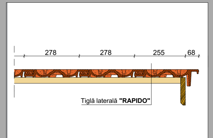
Montaj tigla laterala dreapta
